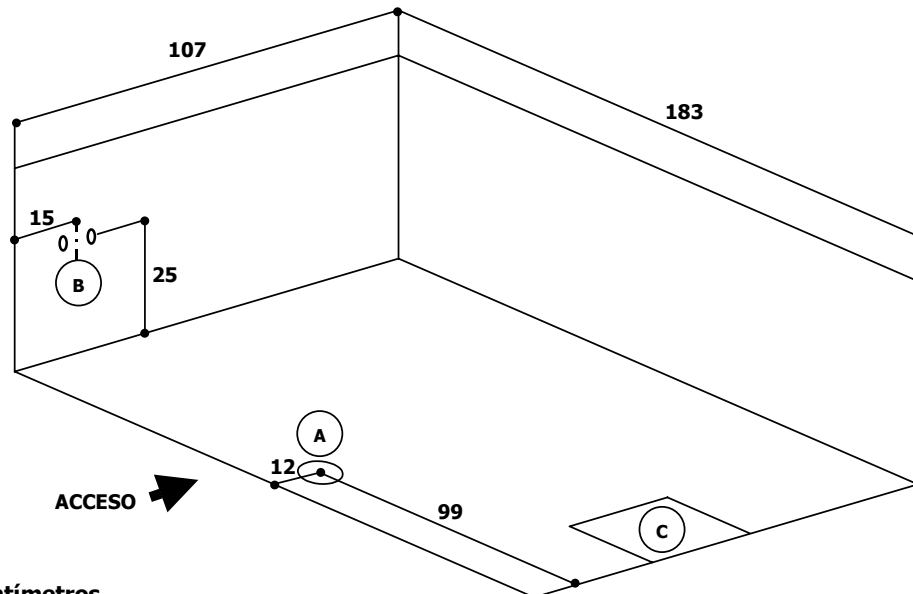
Figura 1: Conjunto Desagüe Rebalse Remoto.
