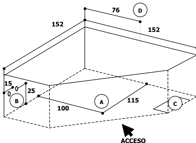
Figura 1: Conjunto Desagüe Rebalse Remoto.
